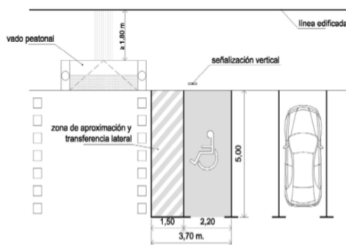
Figura 2. Plaza de aparcamiento reservada con acceso desde paso de peatones
