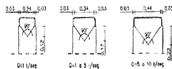
CHAPAS VERTEDERO
