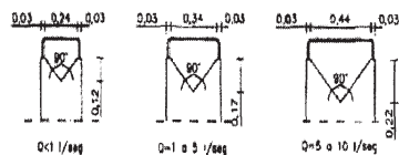
CHAPAS VERTEDERO
